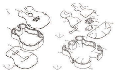
設計した楽器構造
