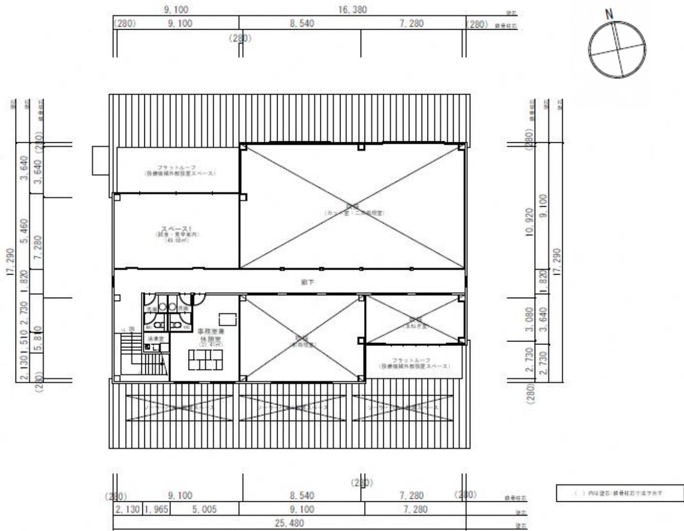
2階平面図 2階床面積：154.02㎡
