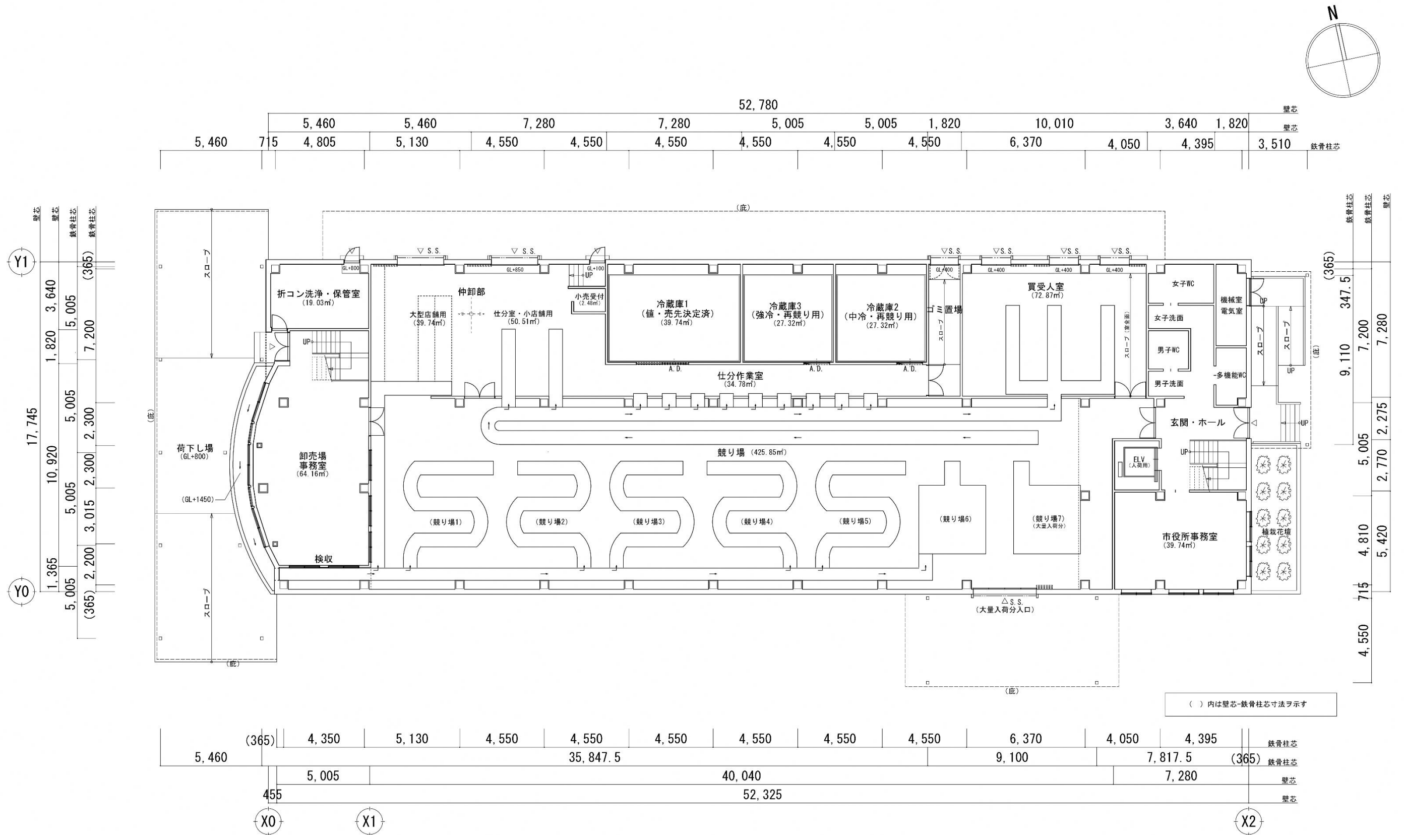
1階平面図
