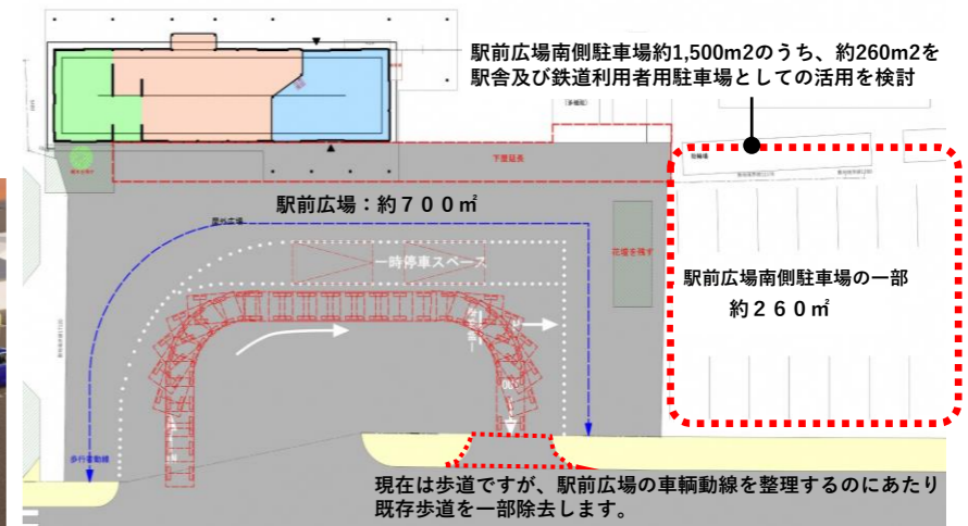
駅前広場配置計画図
