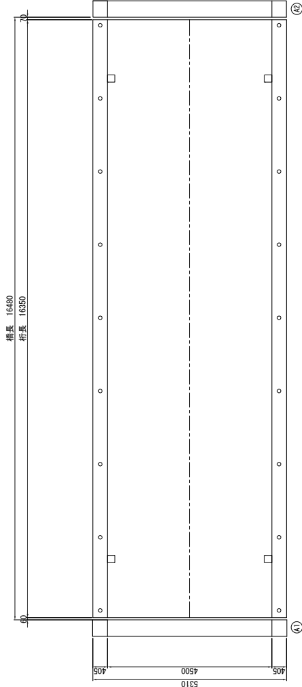
平面図 S=1:50
