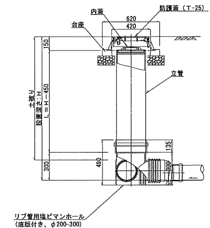
横断面図
