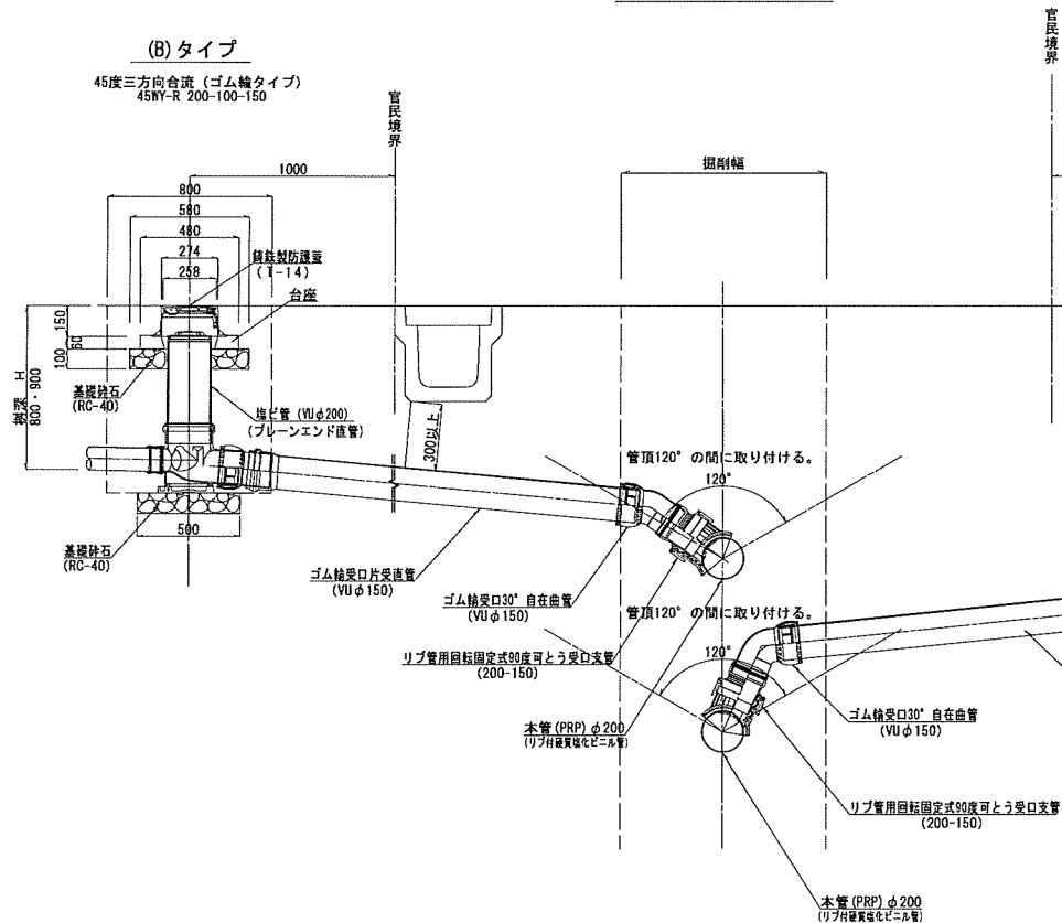
断面図
