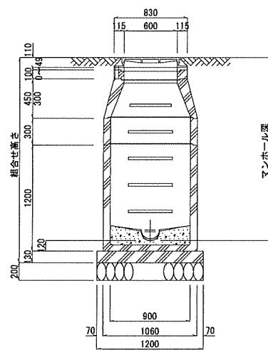
縦断面図
