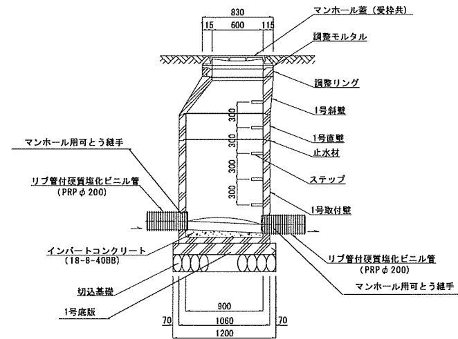
横断面図
