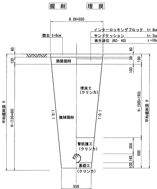
(インターロッキング歩道部)
