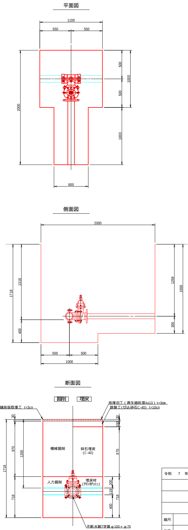
不断水割T字管設置工箇所 φ 100 × φ 75 DP=1.200m
