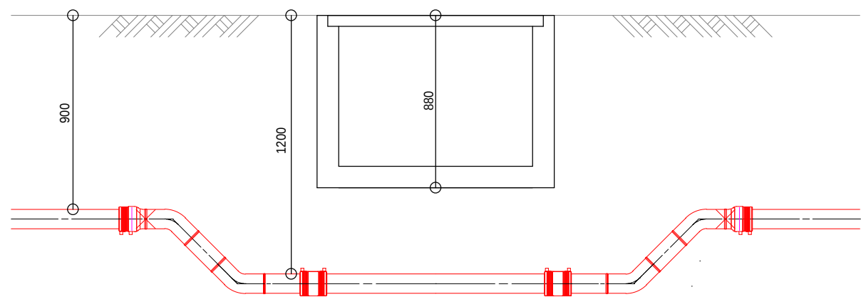
暗渠下越断面図
