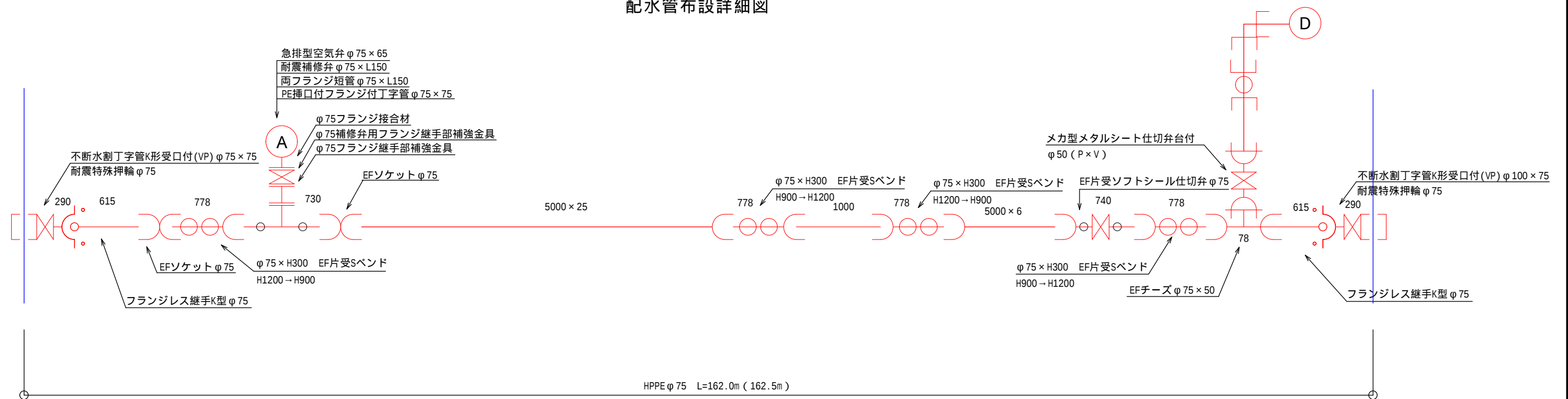
配水管布設詳細図
