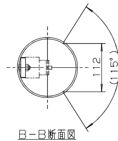
B-B断面図
