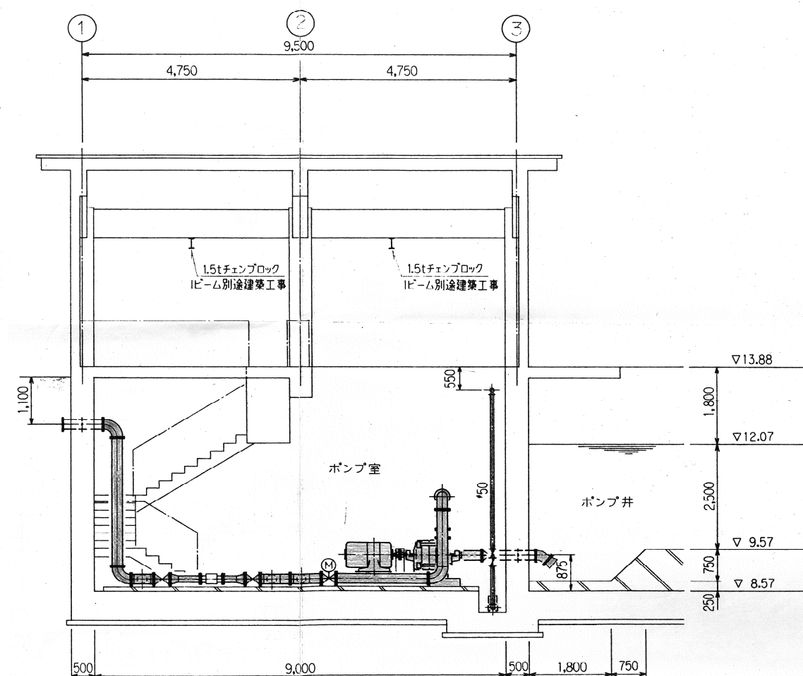
B-B断面図
