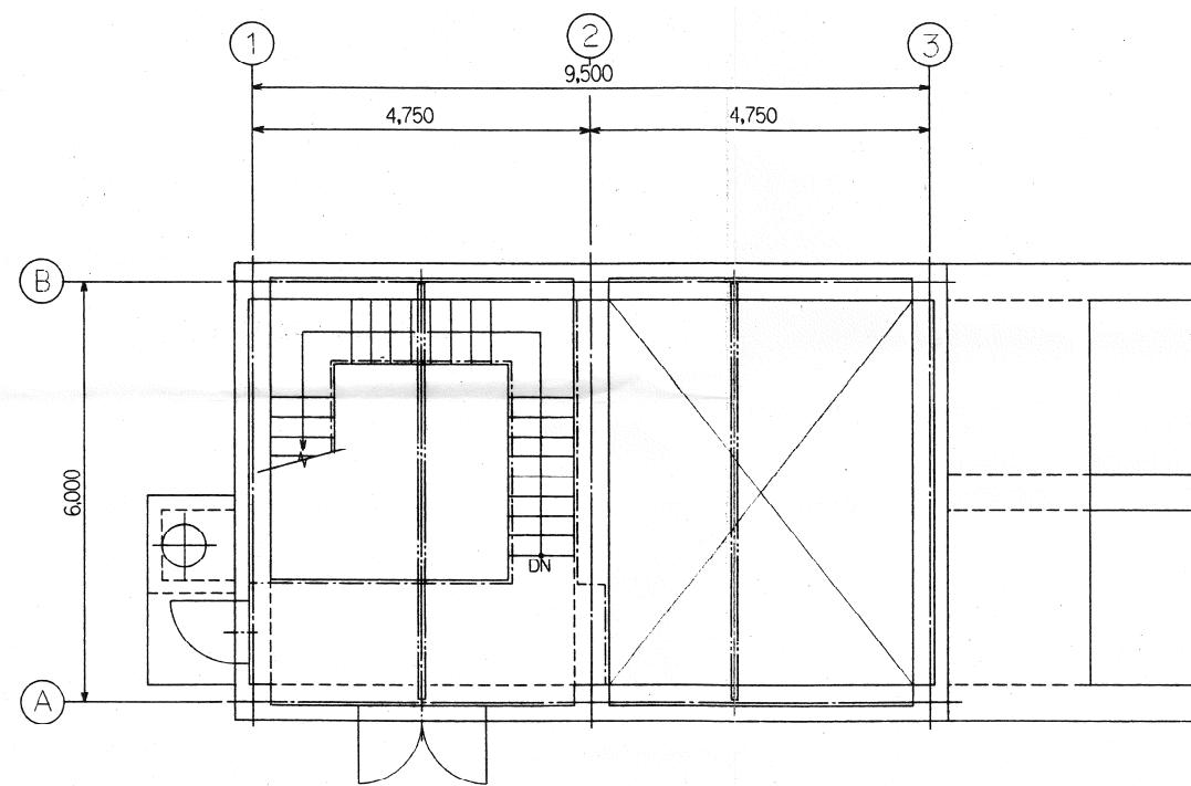
1階平面図
