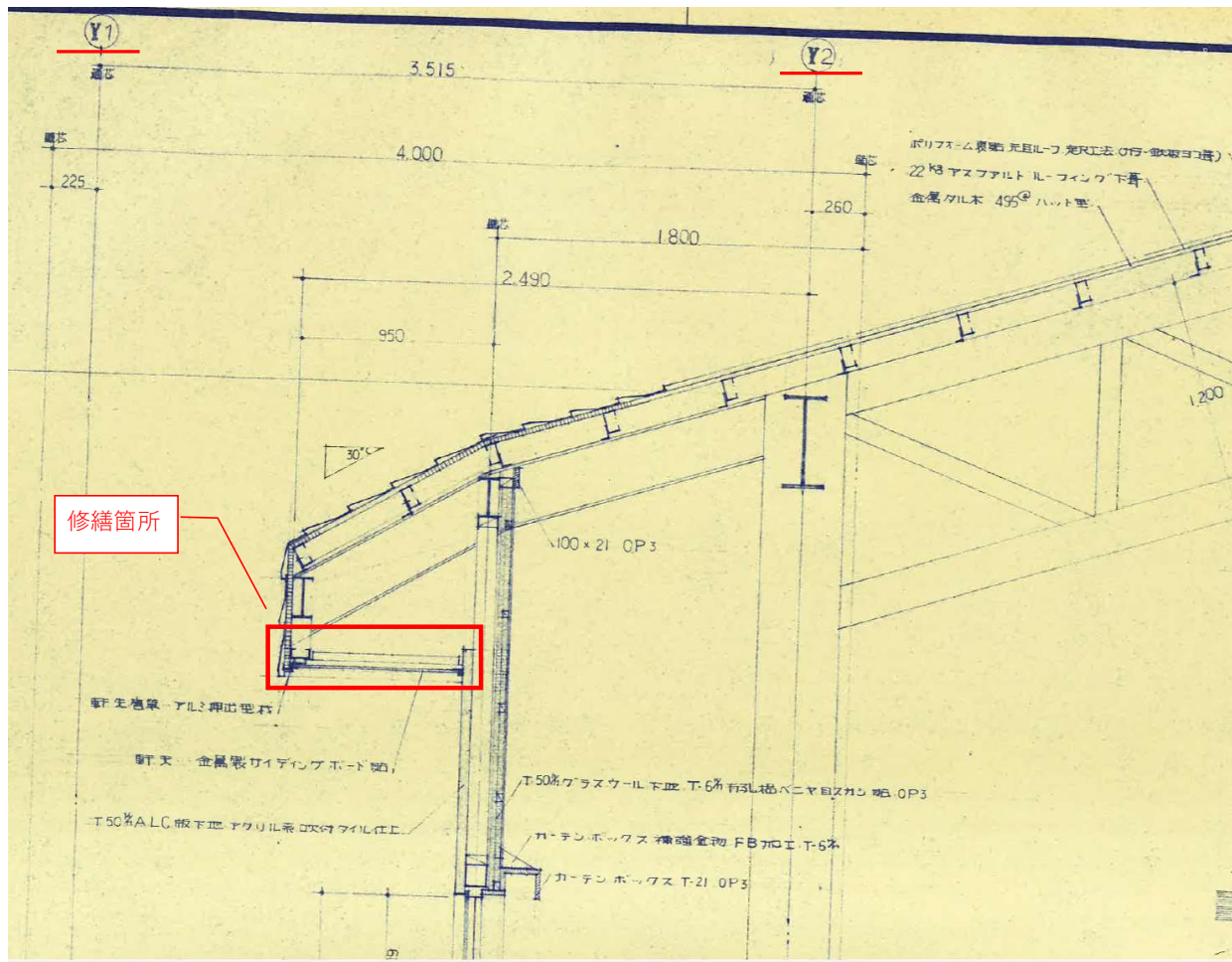
参考図（矩計図）
