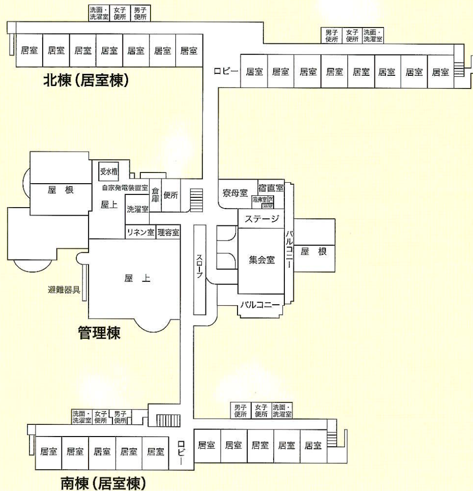
【2F平面図】
