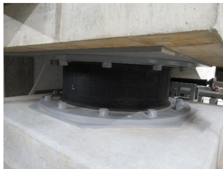
免震構造（福島市役所）
