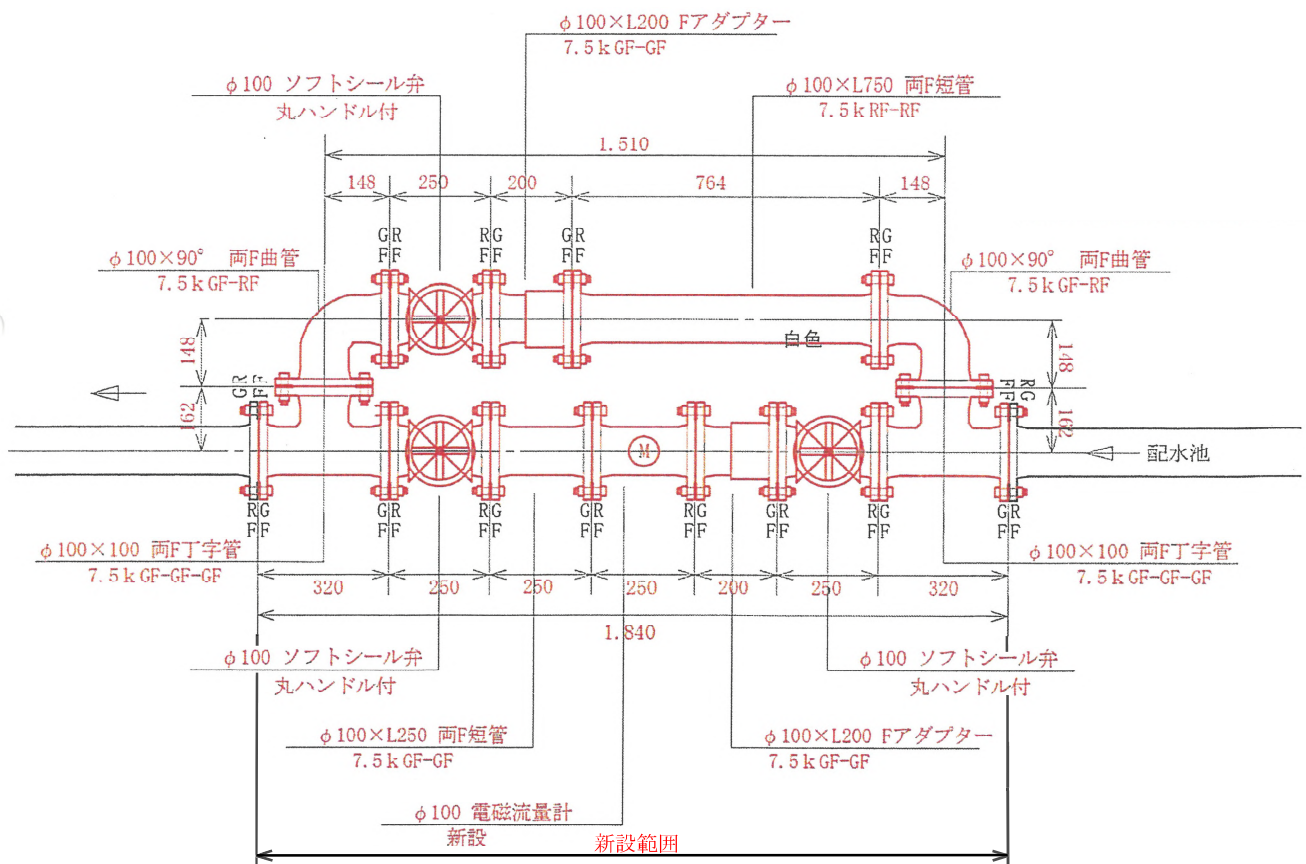
新設図 (更新後) S=NON
