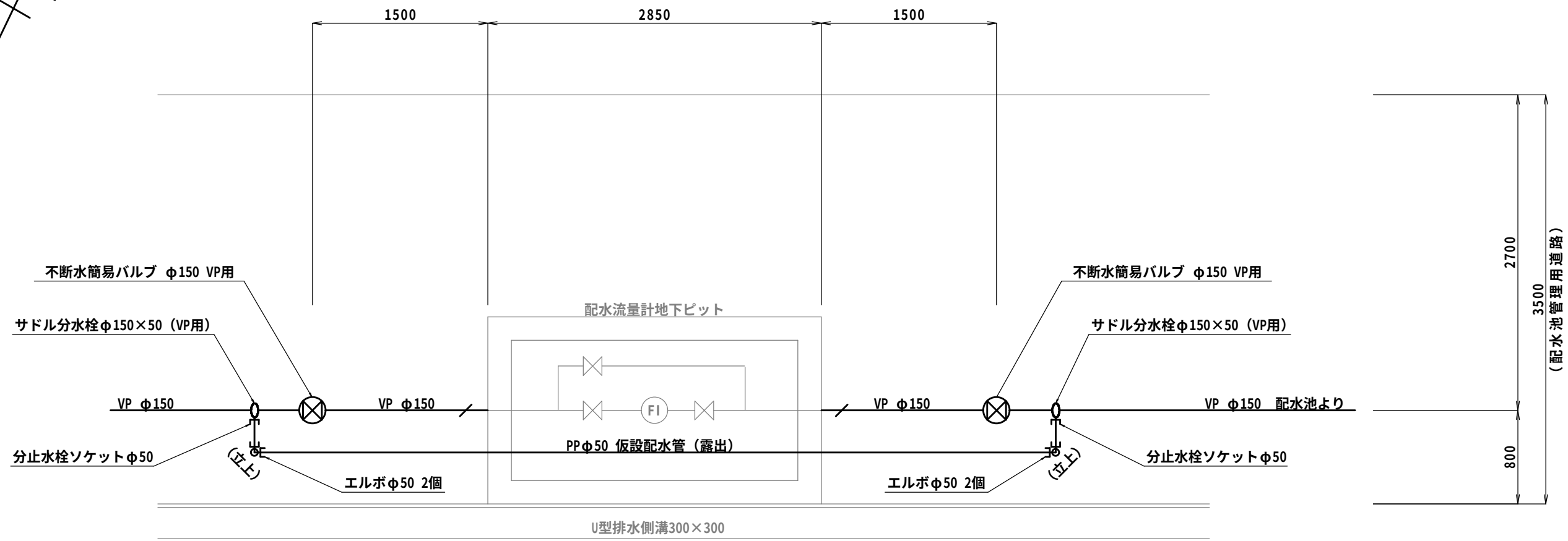
施工範囲平面図 S=1:20
