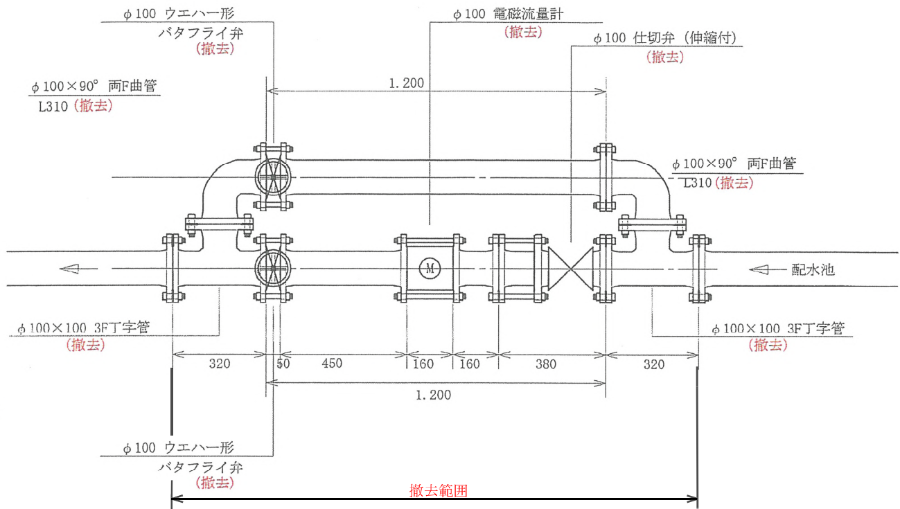
撤去図 (更新前) S=NON
