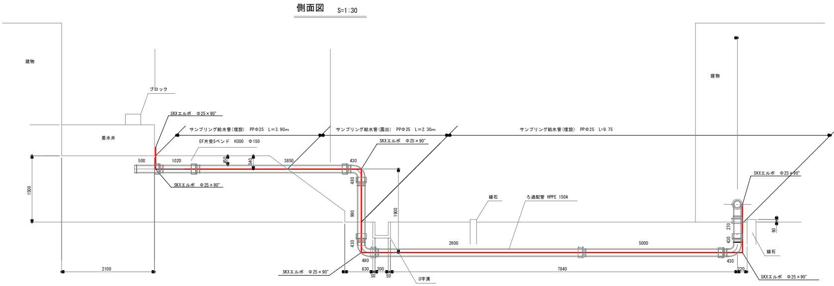
側面図 S=1:30
