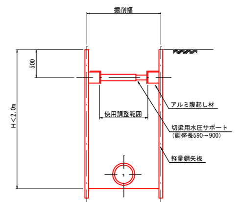
支保1段 断面図
