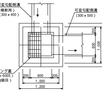
1号横断溝作業土工
