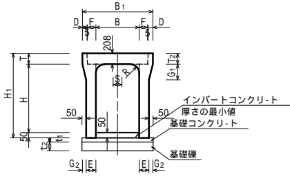
可変勾配側溝 (縦断用) NON SCALE
