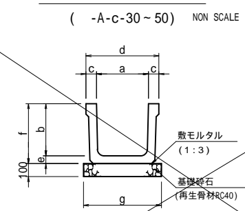
U型側溝 (-A-c-30~50) NON SCALE
