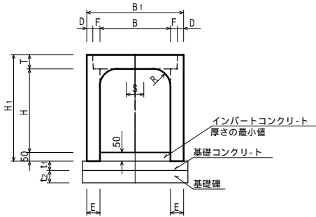
可変勾配側溝 (横断用) NON SCALE
