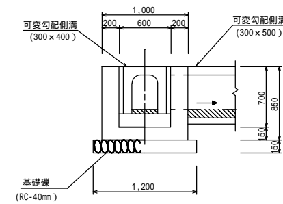
集水樹工 ②タイプ S=1:30
