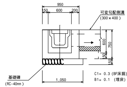
集水樹工 ①タイプ 1.0基当り
