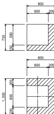
既設樹工取壊し(A) S=1:30
