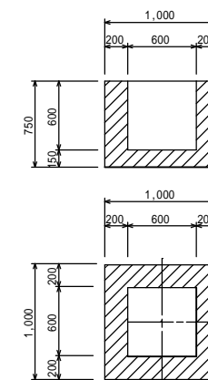
既設樹工取壊し(B) S=1:30
