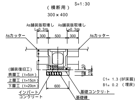
可変勾配側溝 (横断用) S=1:30
