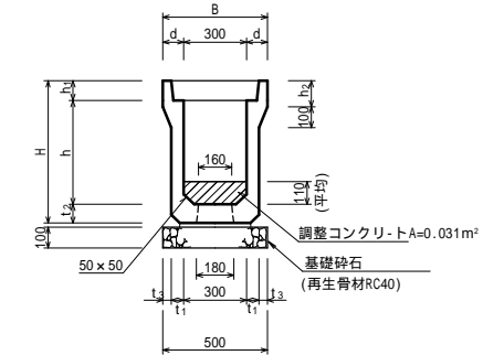
新設勾配側溝 (縦断用) NON SCALE
