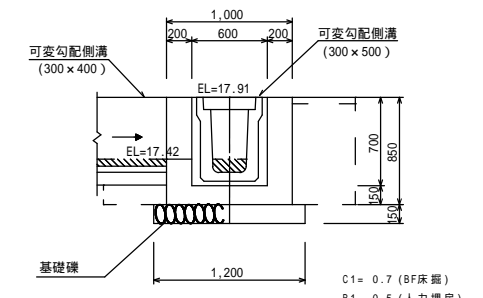
集水樹工 ②タイプ S=1:30
