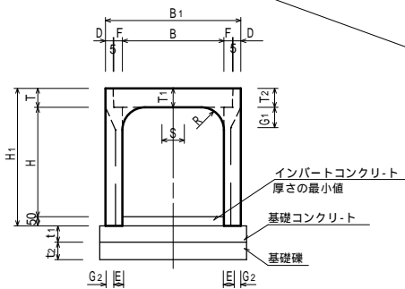
可変勾配側溝 NON SCALE (縦断用横断用)
