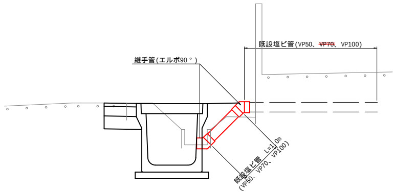
断面図
