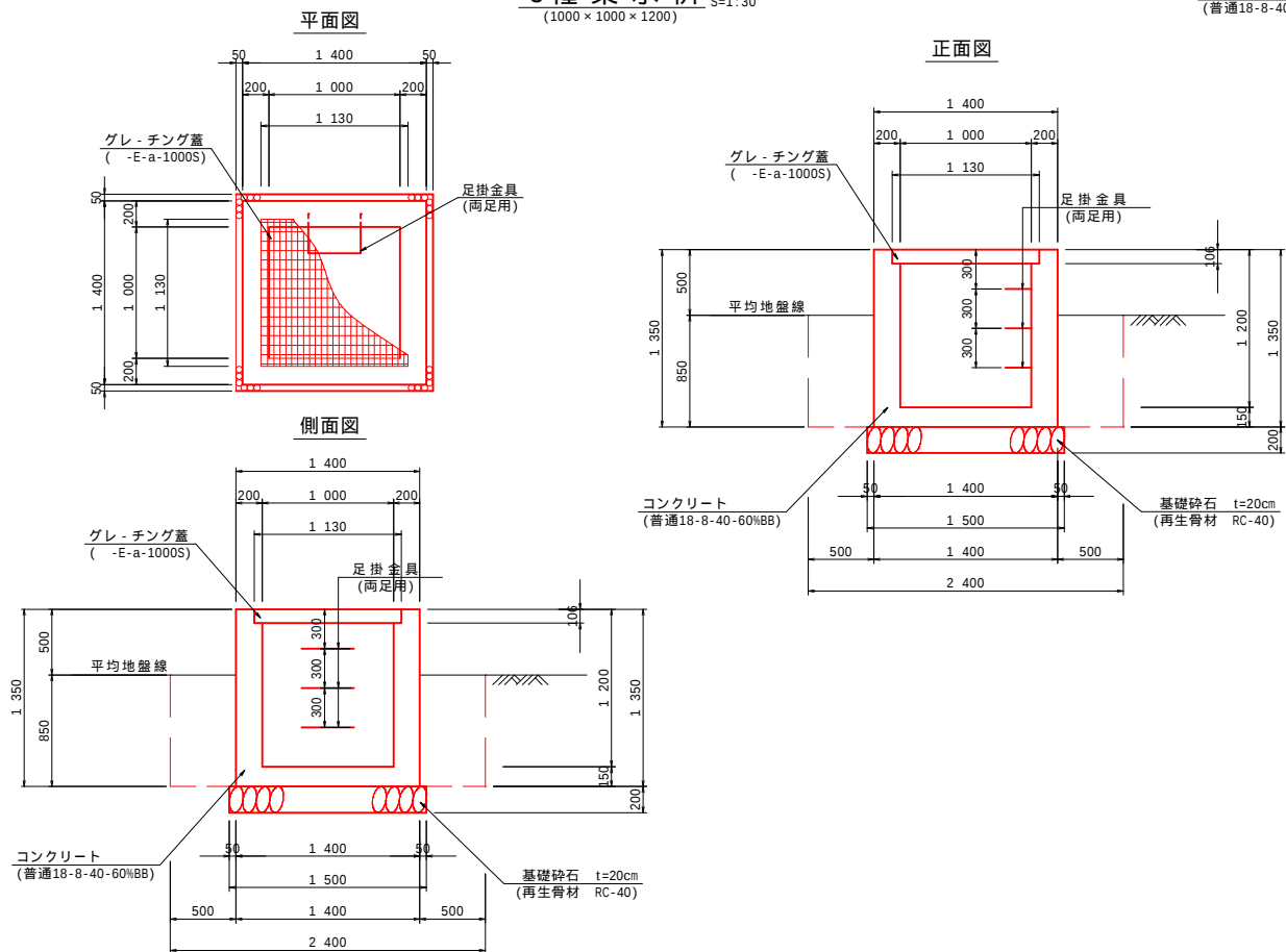
3種集水枡 S=1:30 (1000×1000×1200)
