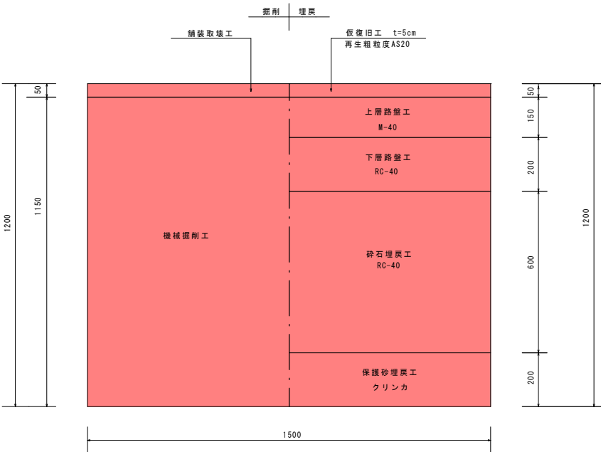
試掘土工（市道）車道舗装部 L1.5m×W1.5m×H1.2m
