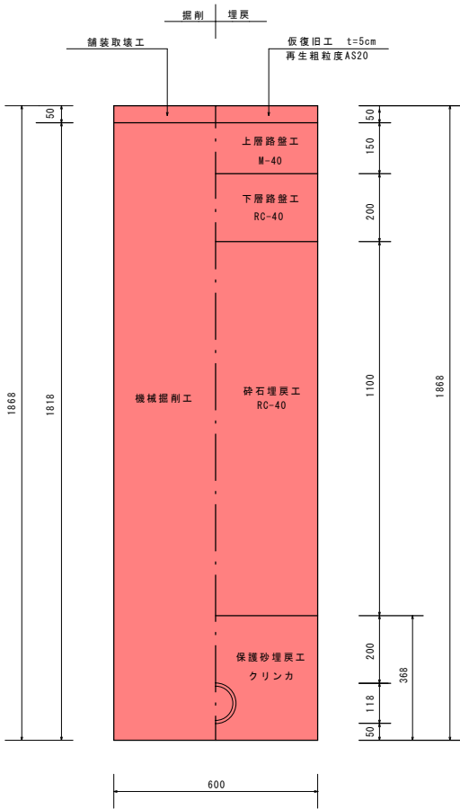
土工③（市道）車道舗装部 DIP-NS（E種管）φ100 DP=1.7m
