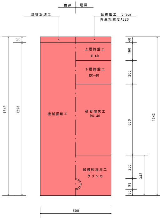
土工⑤（市道）車道舗装部 DIP-NS（E種管）φ75 DP=1.2m
