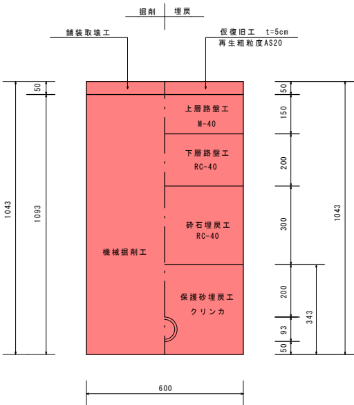
土工④（市道）車道舗装部 DIP-NS（E種管）φ75 DP=0.9m
