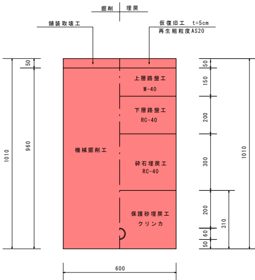
排泥土工①（市道）車道舗装部 HIVPφ50 DP=0.9m
