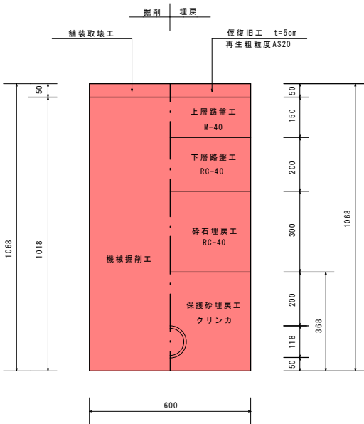
土工①（市道）車道舗装部 DIP-NS（E種管）φ100 DP=0.9m
