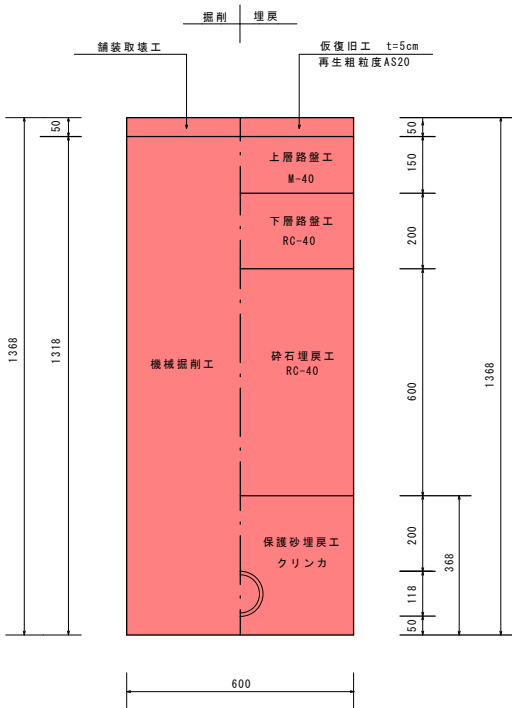
土工②（市道）車道舗装部 DIP-NS（E種管）φ100 DP=1.2m
