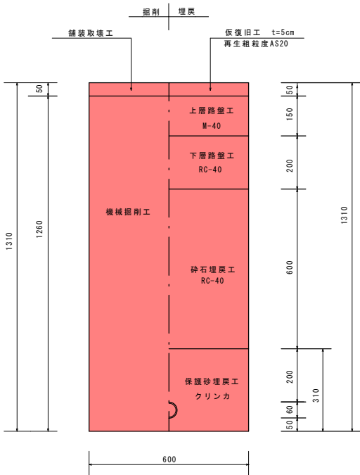
排泥土工②（市道）車道舗装部 HIVPφ50 DP=0.9m
