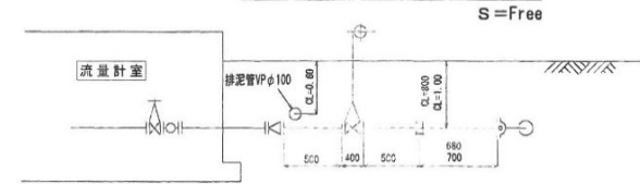
配管詳細図(断面図)
