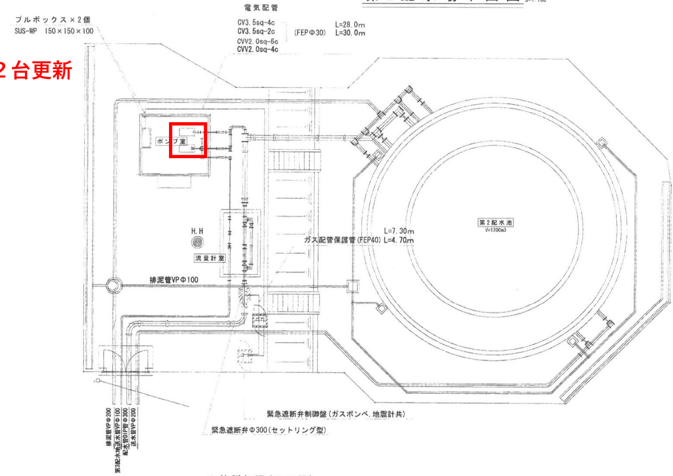
配管詳細図(平面図)
