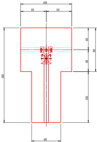
側面図
