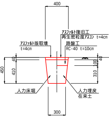
給水管宅内部土工 (アスファルト部, H=0.45) S=1:20
