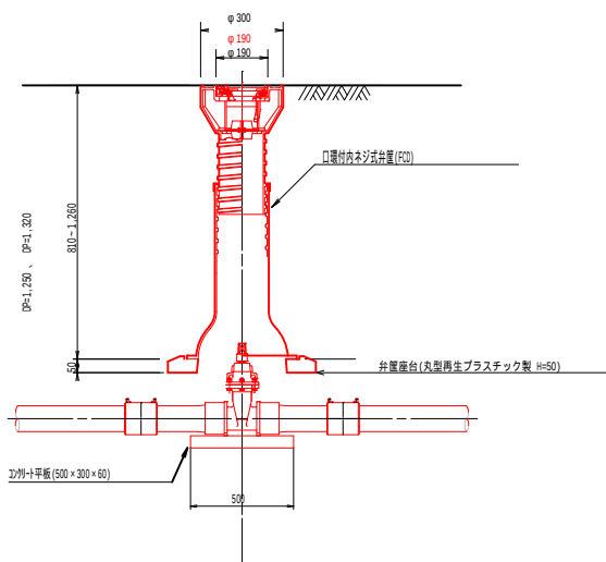
断面图
