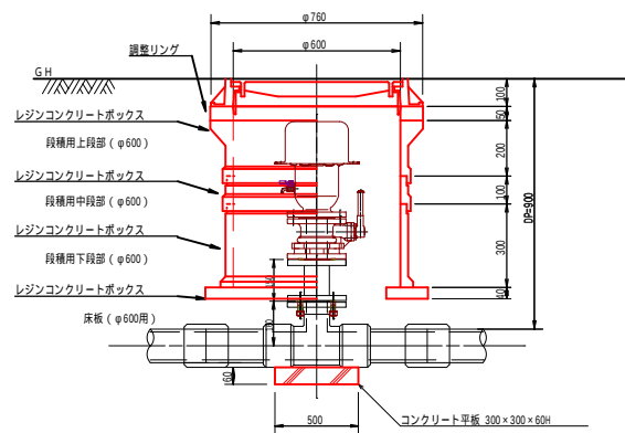
断面图
