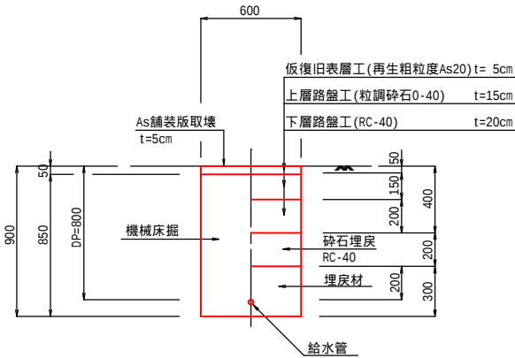
給水管市道部土工 (アスファルト部, H=0.90) S=1:20
