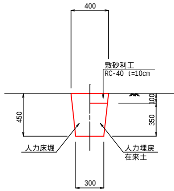
給水管宅内部土工 (在来土部, H=0.45) S=1:20
