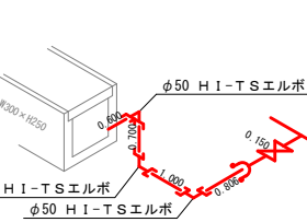
φ50 排泥管詳細図-4
