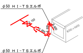
φ50 排泥管詳細図-4
