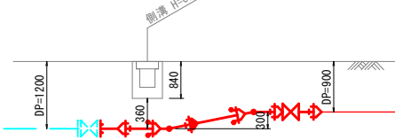
e-e 断面図
