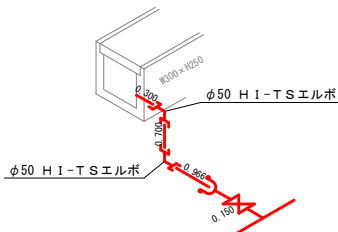
φ50 排泥管詳細図-1
