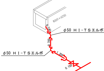
φ50 排泥管詳細図-3
