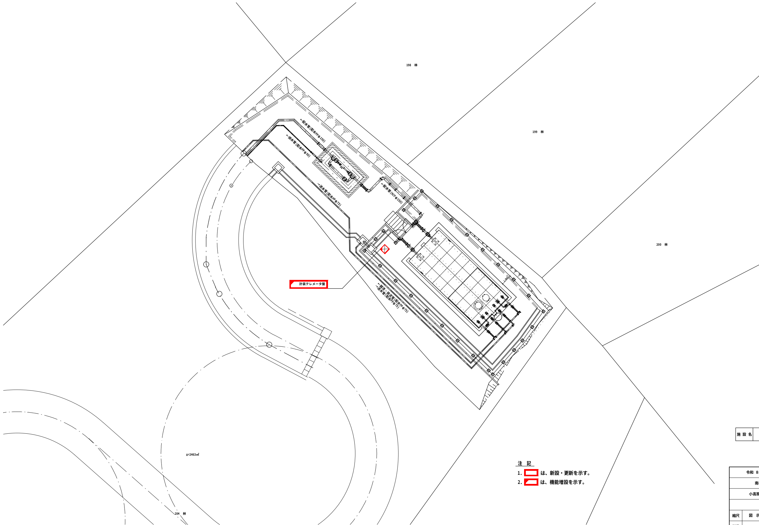
北部第2配水池 平面図 S=1:100
