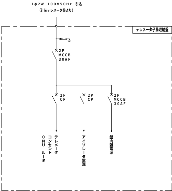
単線接続図
