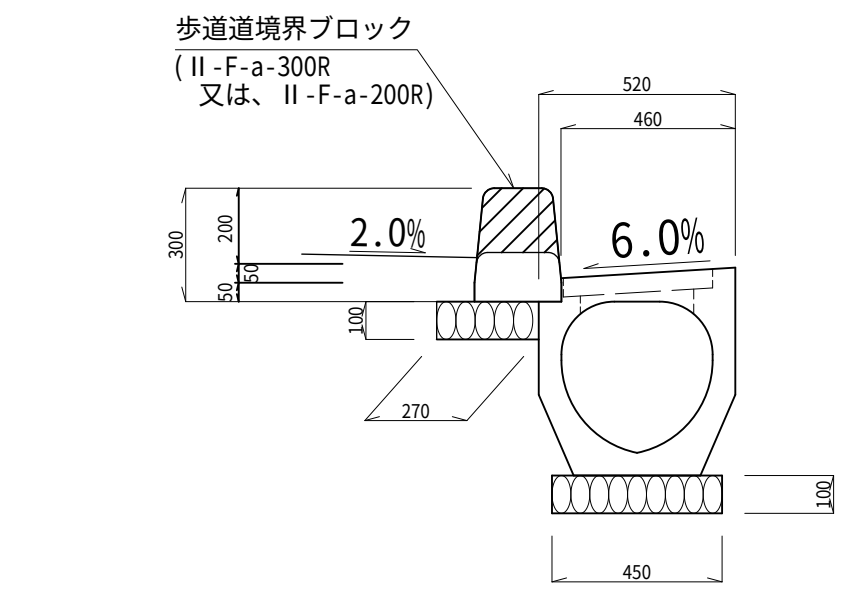
歩道境界ブロック材料表(10m当り)
