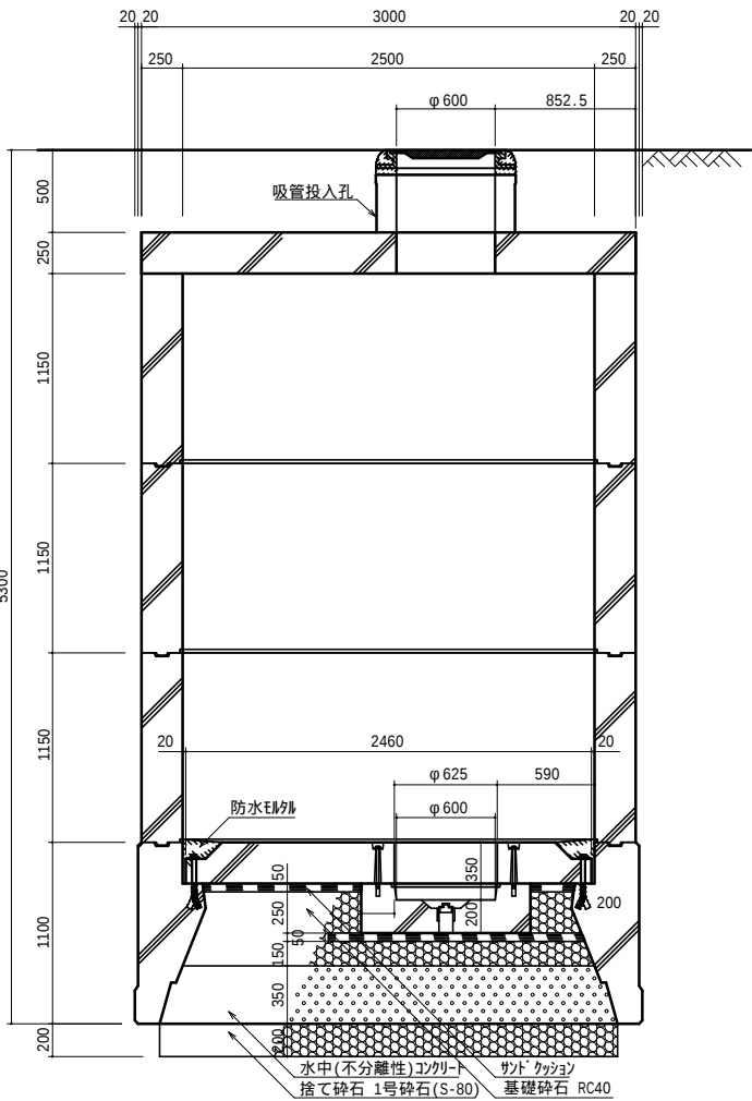
C - C 断面図 S=1:50
