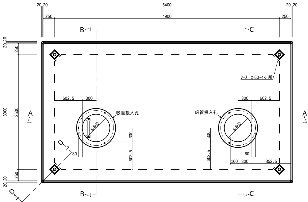
平面図 S=1:50
