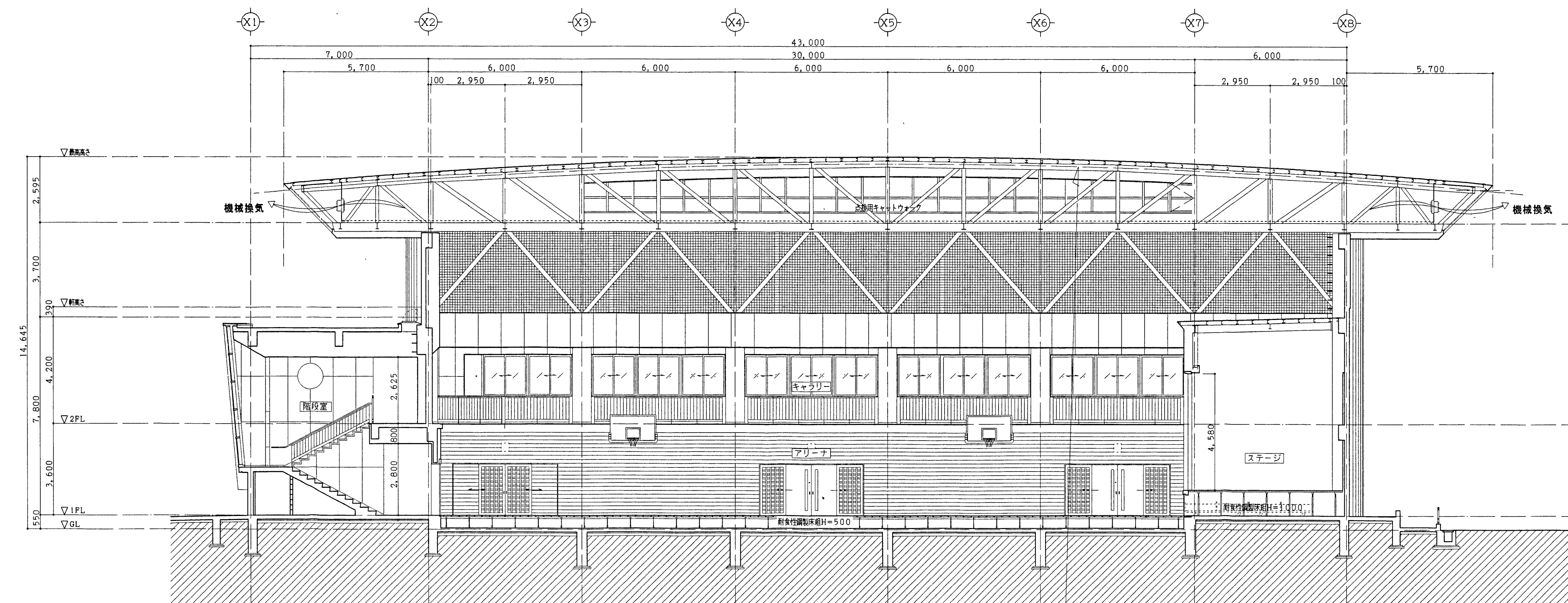
南-北断面図 S=1:100
