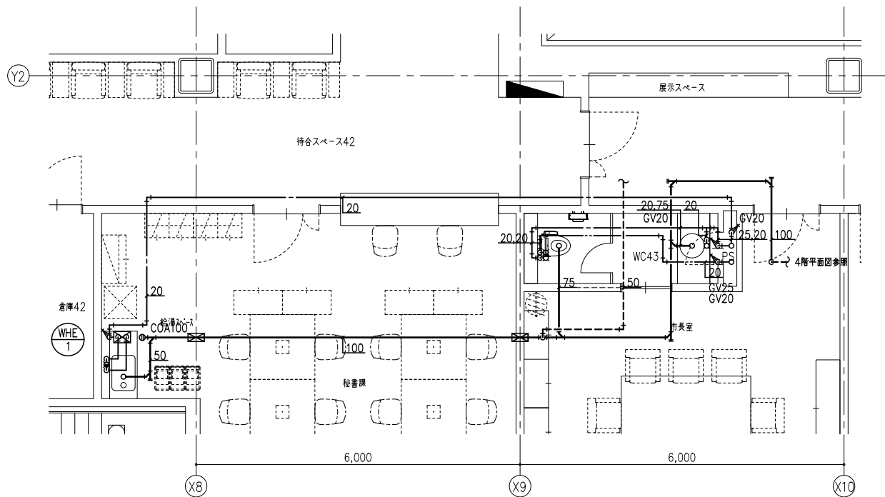
4階詳細図-2 S=1/50 (A1)
