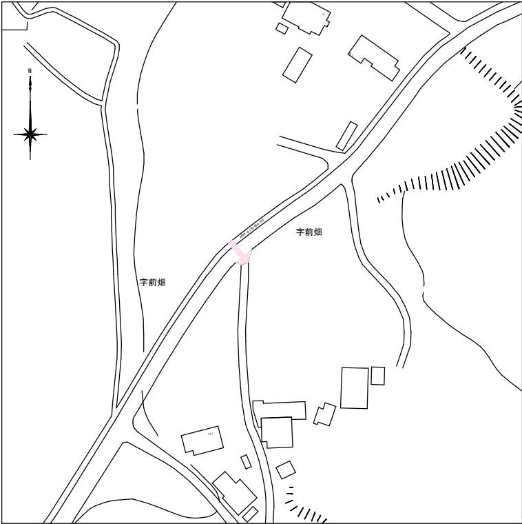
舗装復旧工平面図(5)-1
