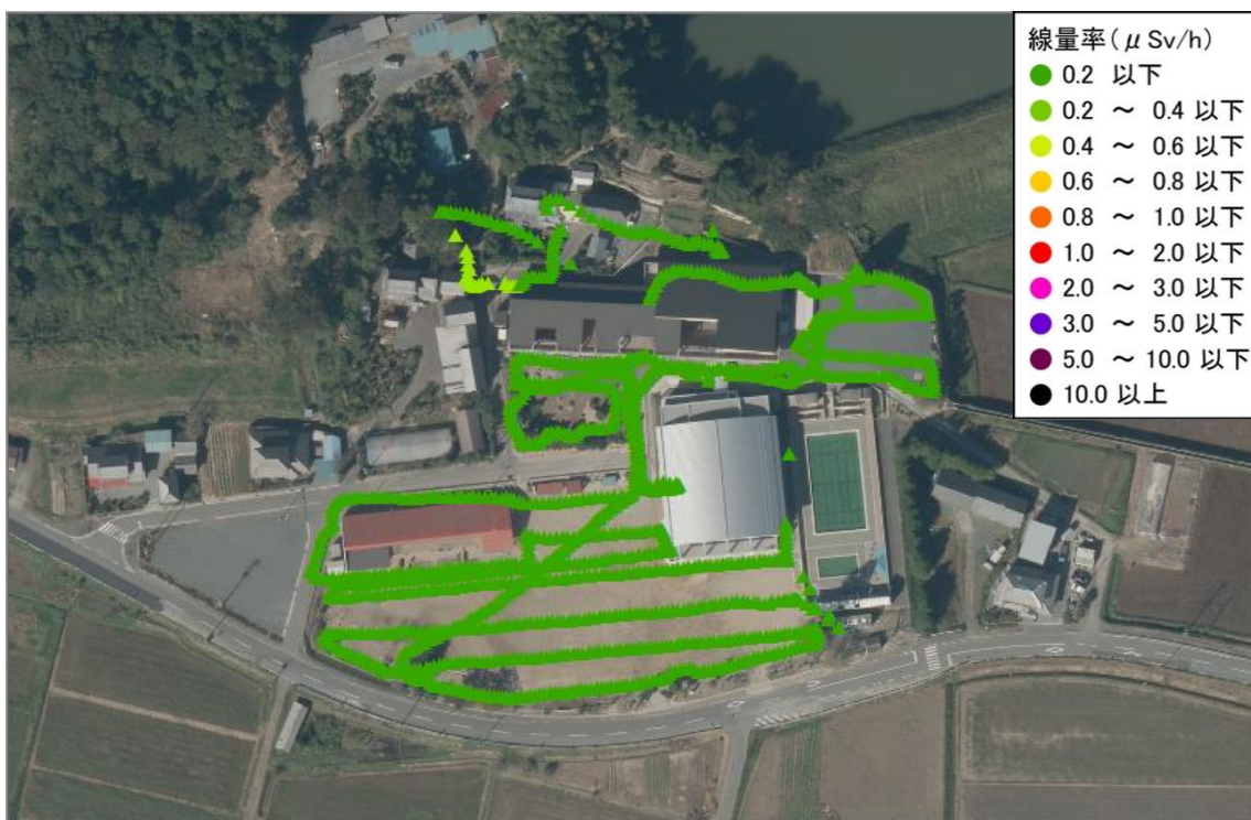
八沢小学校と八沢幼稚園（測定日：2014年6月5日、高さ50cm）
