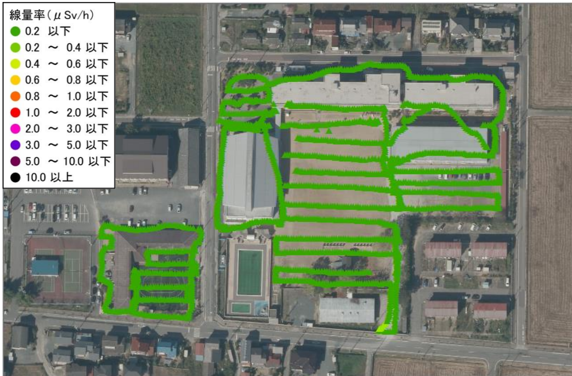
鹿島小学校と鹿島幼稚園（測定日：2014年5月30日、高さ50cm）
