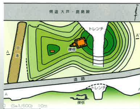
A地区20号墳の測量図
