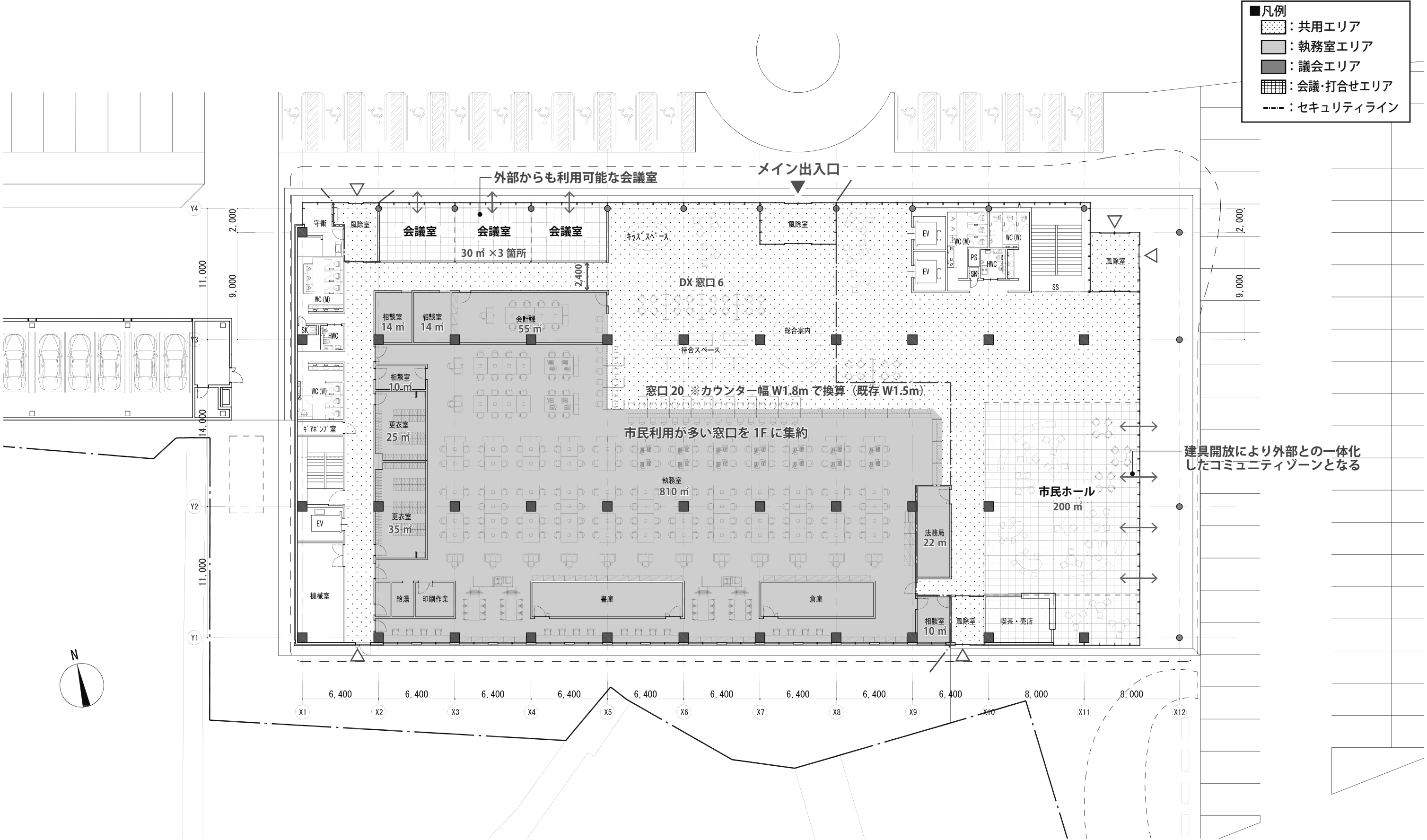
【1階平面図】
