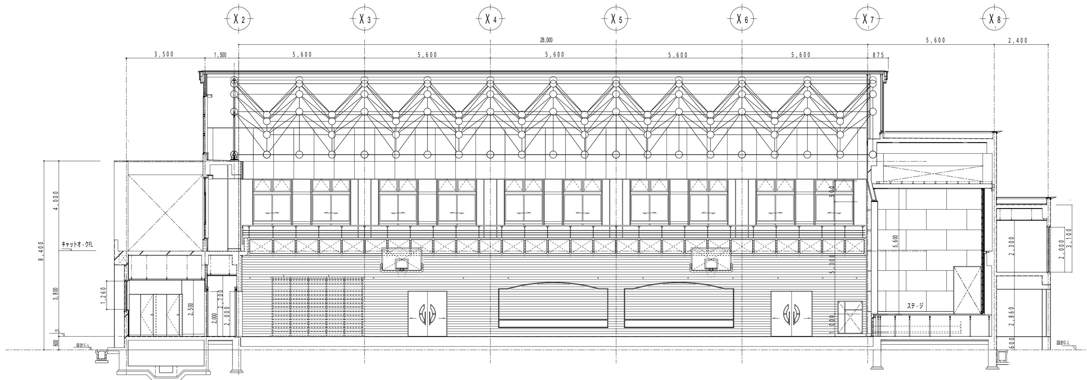
縦断面図 1/100
