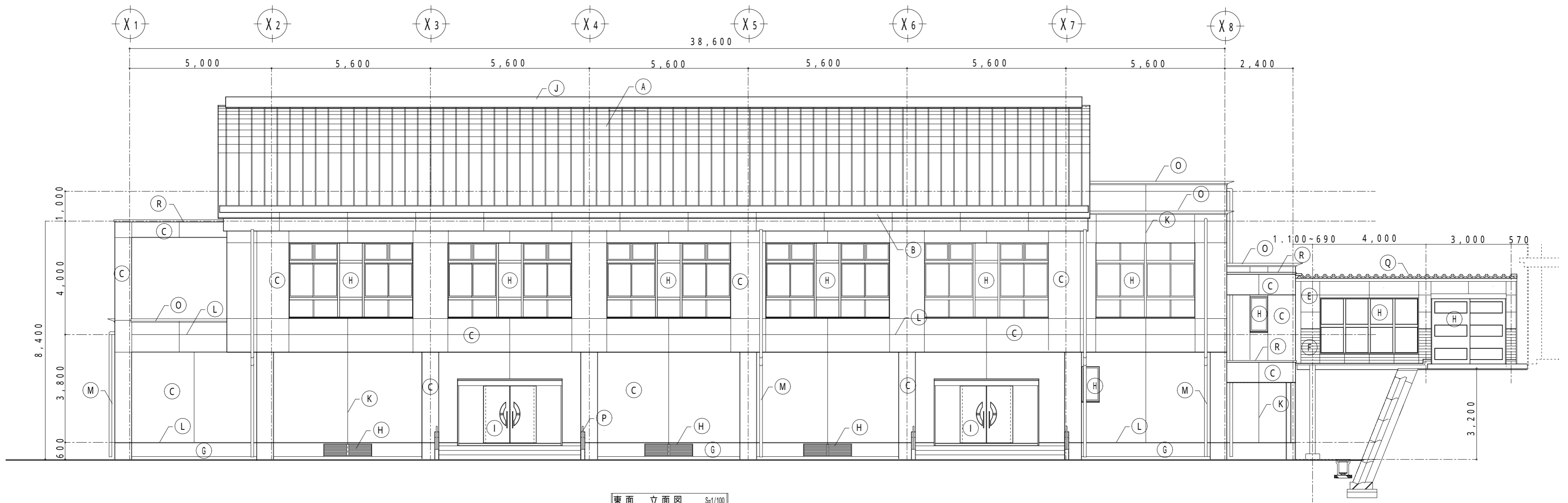
東面 立面图 S=1/100
