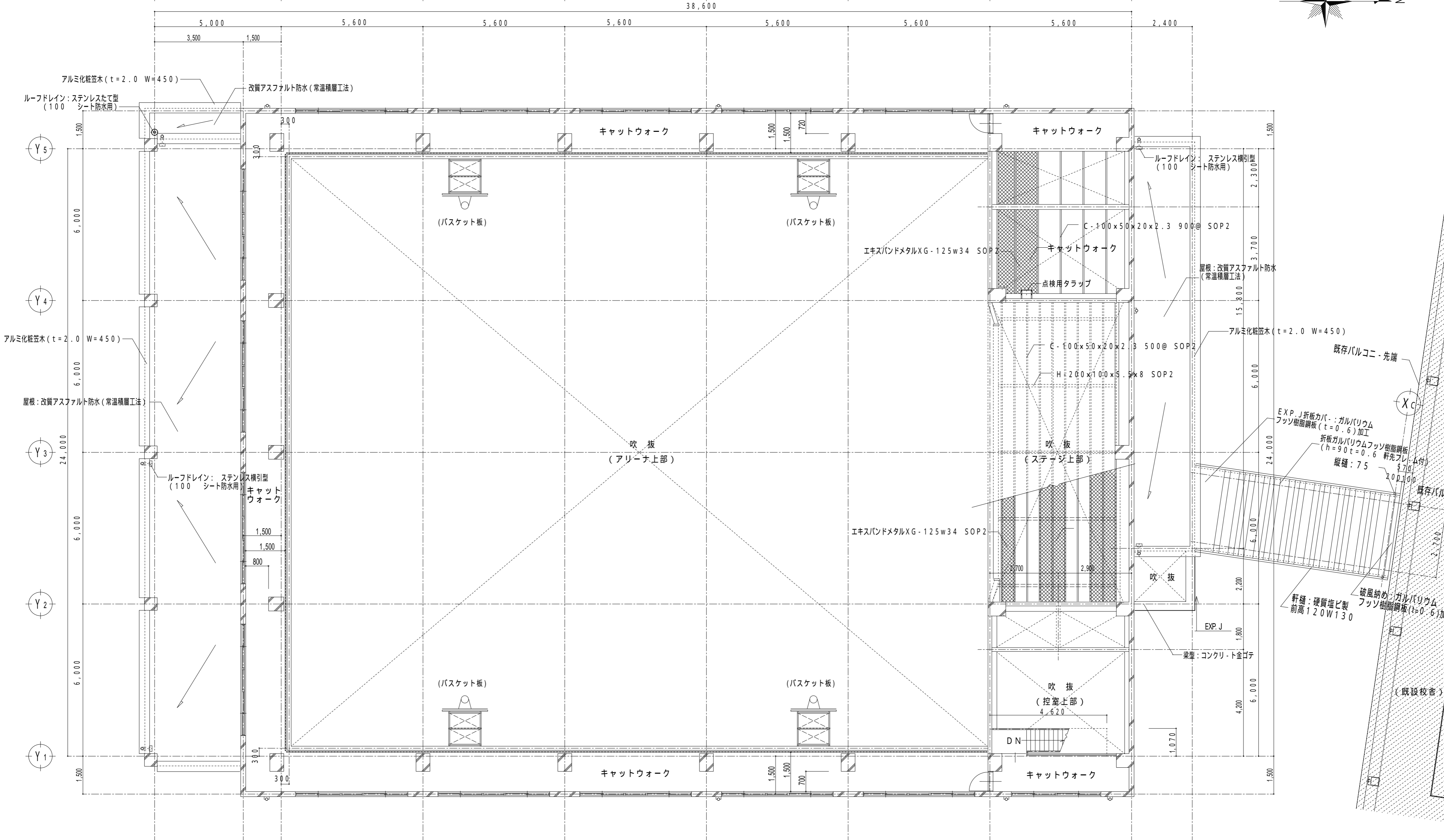
点検用通路 平面図 S=1/100
