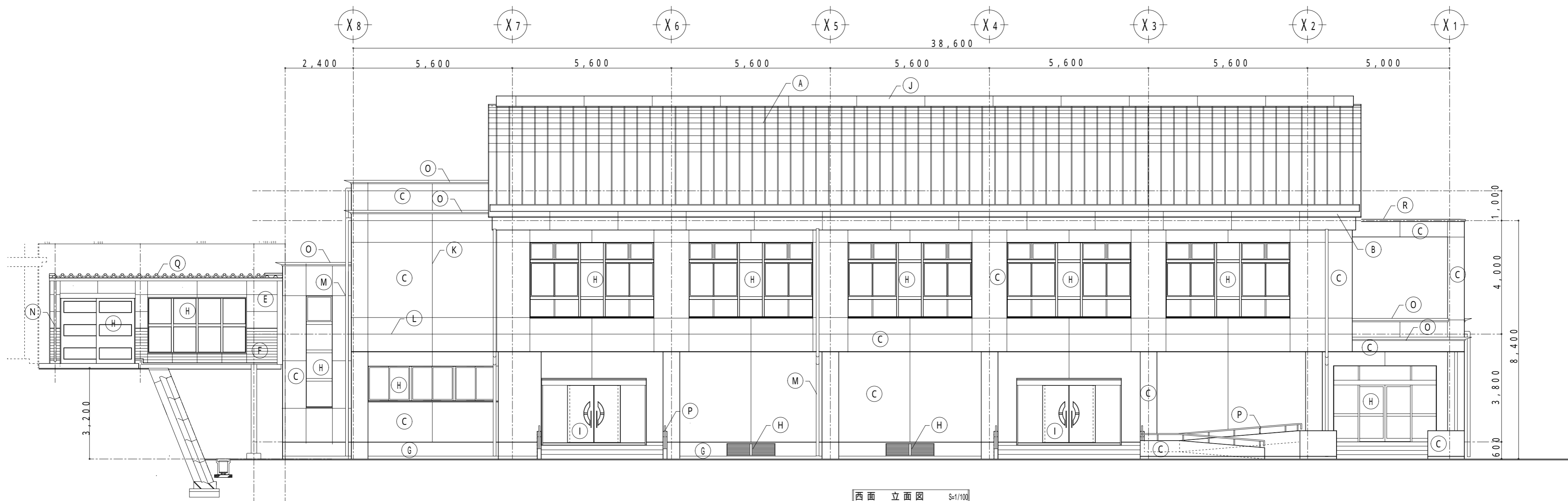
西面 立面図 S=1/100
