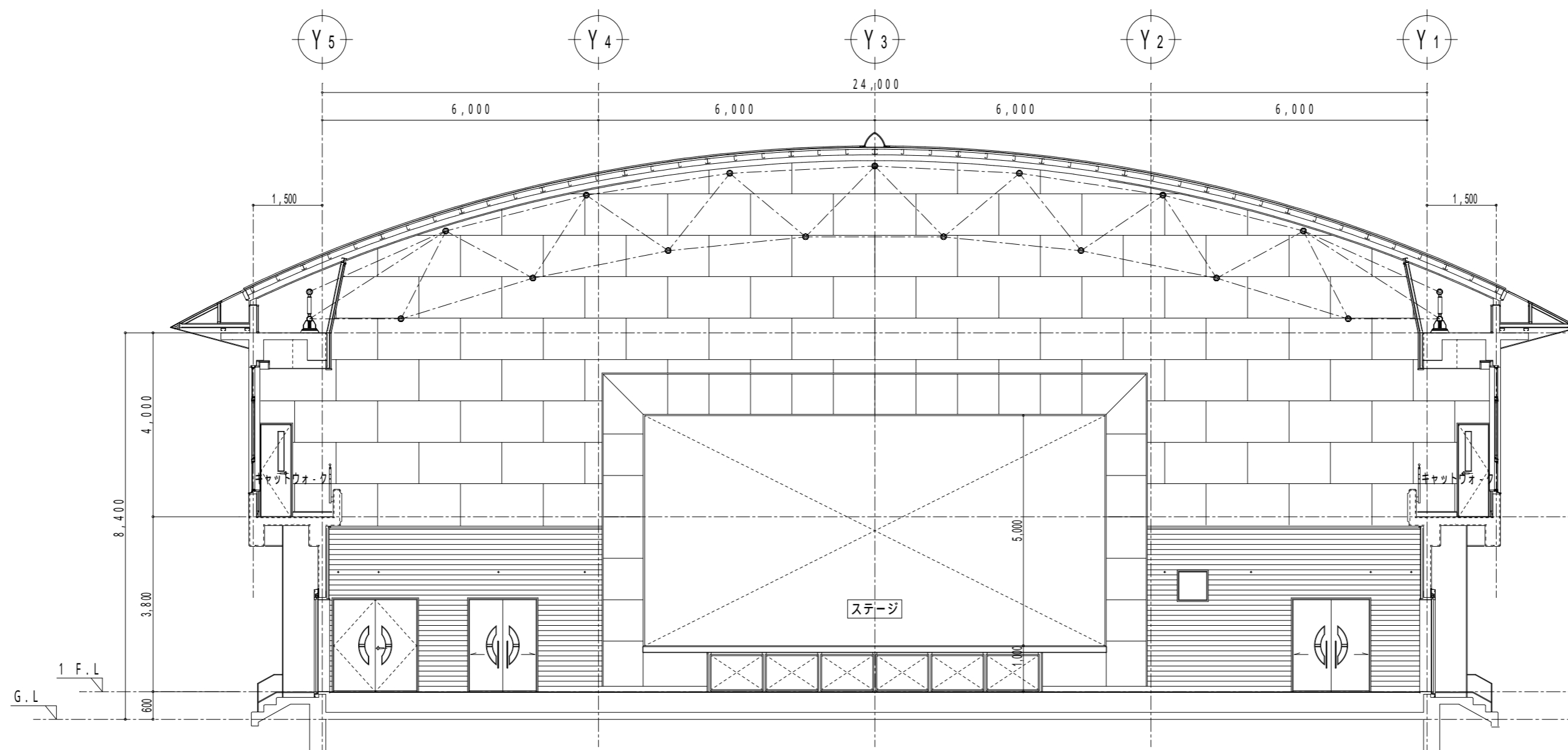
横断面図 1/100
