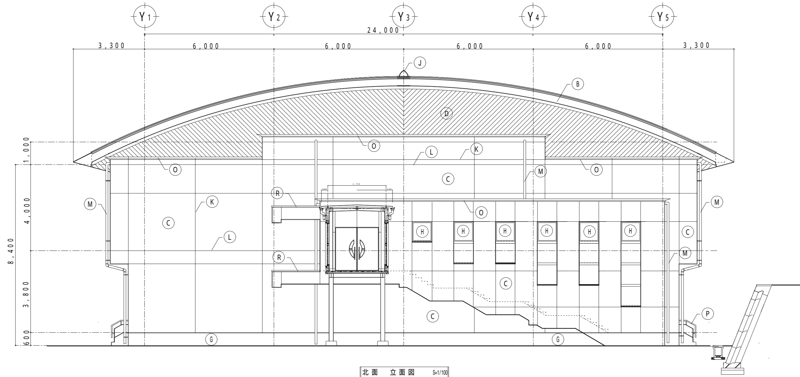
北面 立面图 S=1/100
