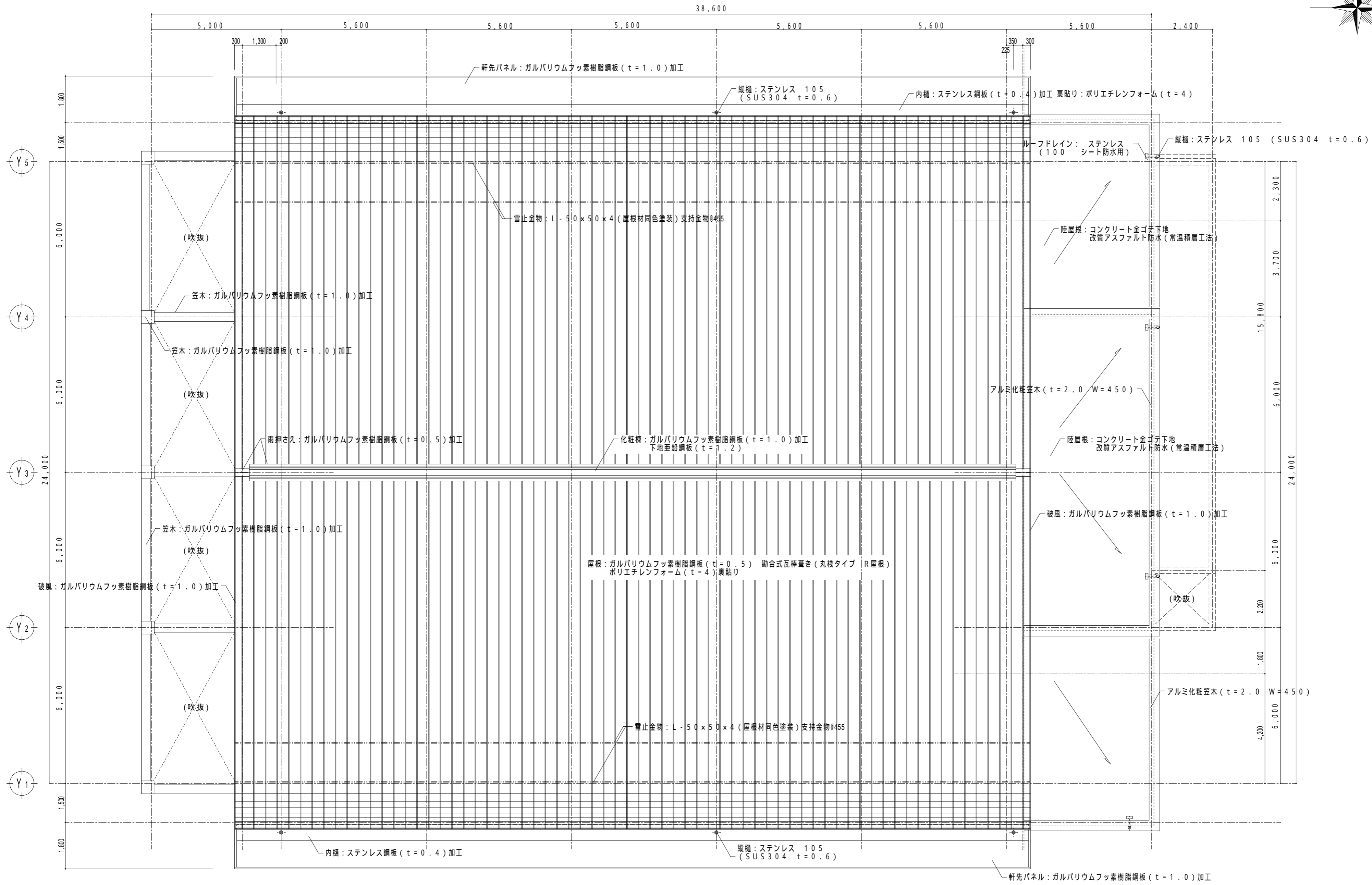
屋根 平面図 S=1/100
